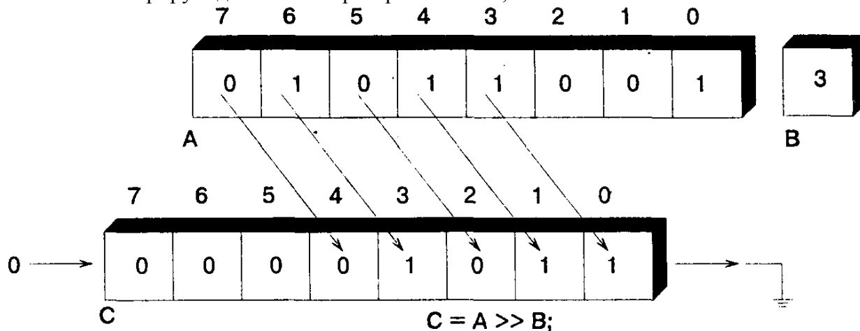
Рисунок 6 – Действия оператора поразрядного сдвига вправо
