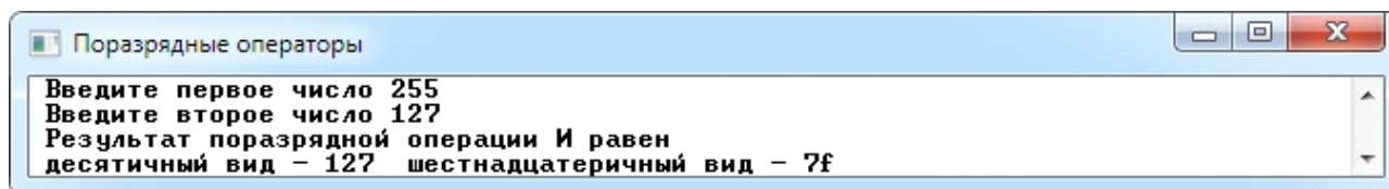
Рисунок 9 – Вариант консольного приложения «Поразрядные операторы»
