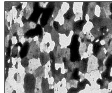
Алюминий отожжённый
