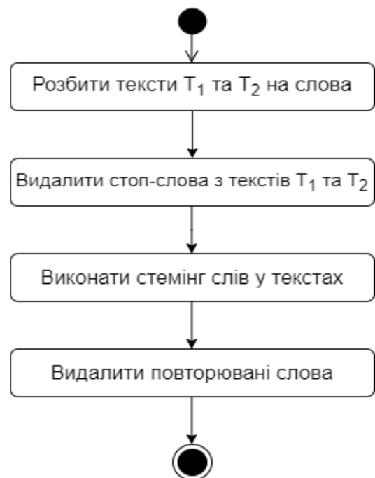
Рис. 1 – Процедура вилучення множин термінів
