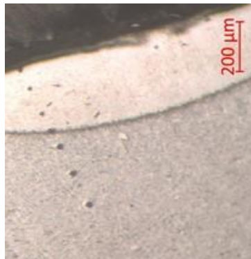
Рис. 1 – Мікроструктура перерізу фрагменту робочої частини різального інструмента, який виготовлений із сталі У8А, після його зміцнення з додатковим застосуванням тертя (х 50)
