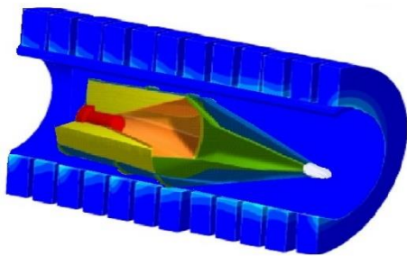
Рис. 1 – Розташування боєприпасу в індукторі
