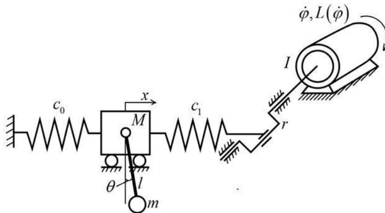
Рис.1. Модель неідеальної системи з маятничовим гасителем коливань
