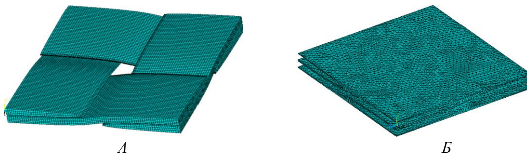
Рис. 1 – Скінчено-елементна модель: а – волокон; б – матриці
