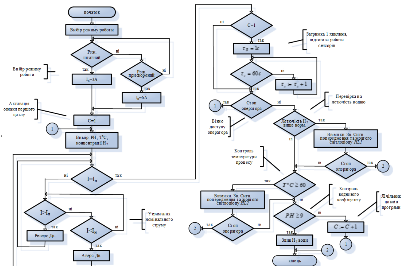
Рисунок 1 – Алгоритм роботи АГВВ
