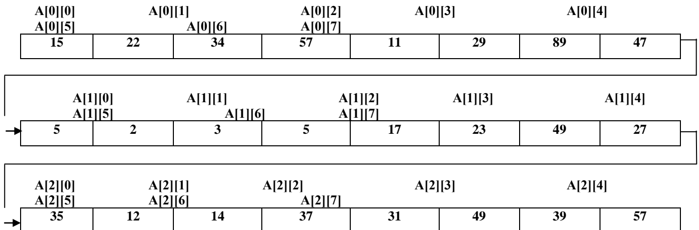
Рис. 1. Значения и расположение в памяти элементов массива A[3][8]
