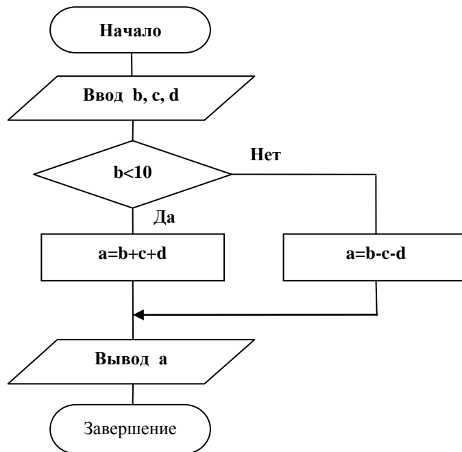
Рис. 2. Блок-схема алгоритма определения переменной a (простые операторы)
