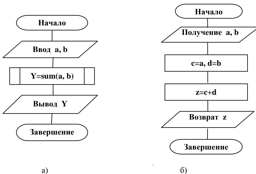
Рис. 3. Блок-схема алгоритма вычисления Y по формуле Y=a+b с использованием функции: а) основная программа; б) функция sum(double c, double d)
