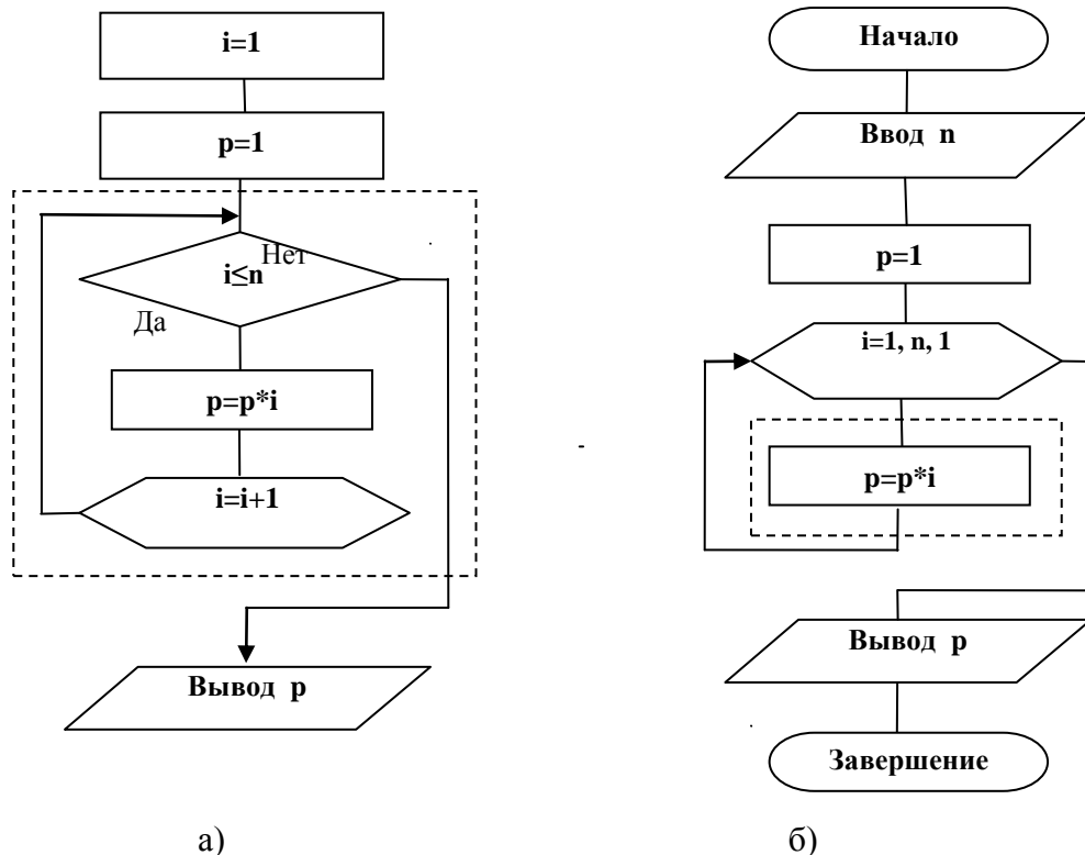
Рис. 4. Блок-схемы вычисления факториала целого числа n : а) вычислительного процесса; б) алгоритма с использованием оператора for
