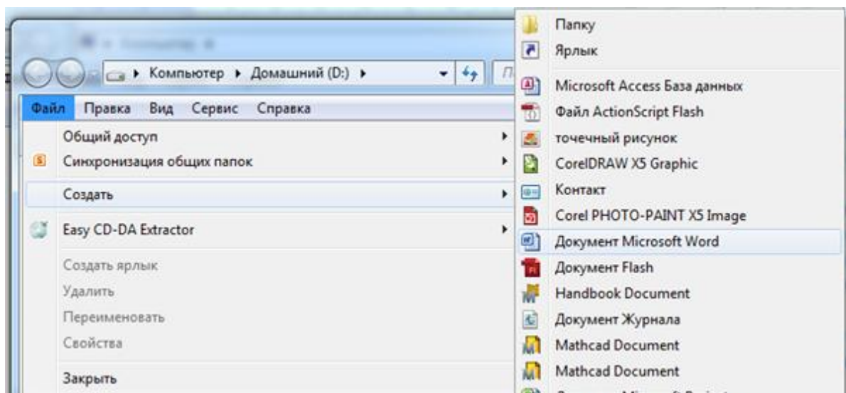
Рис. 6.3 – Створення об'єктів
