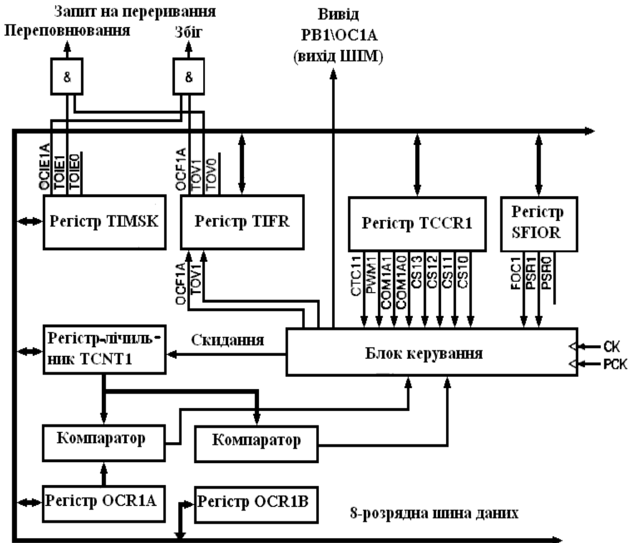
Рисунок 11.2 – Структурна схема таймера T1
