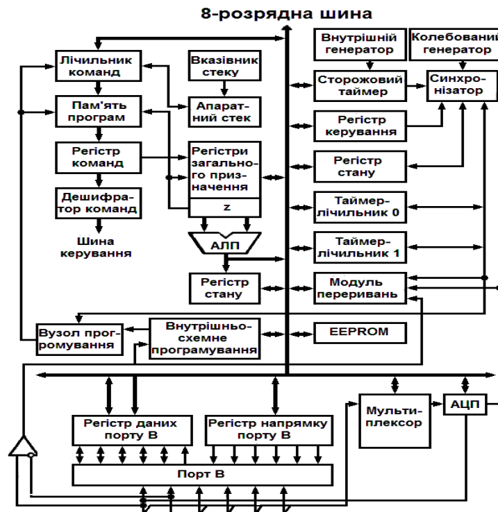
Рисунок 3.2 – Розширена структурна схема мікроконтролера ATtiny15L
