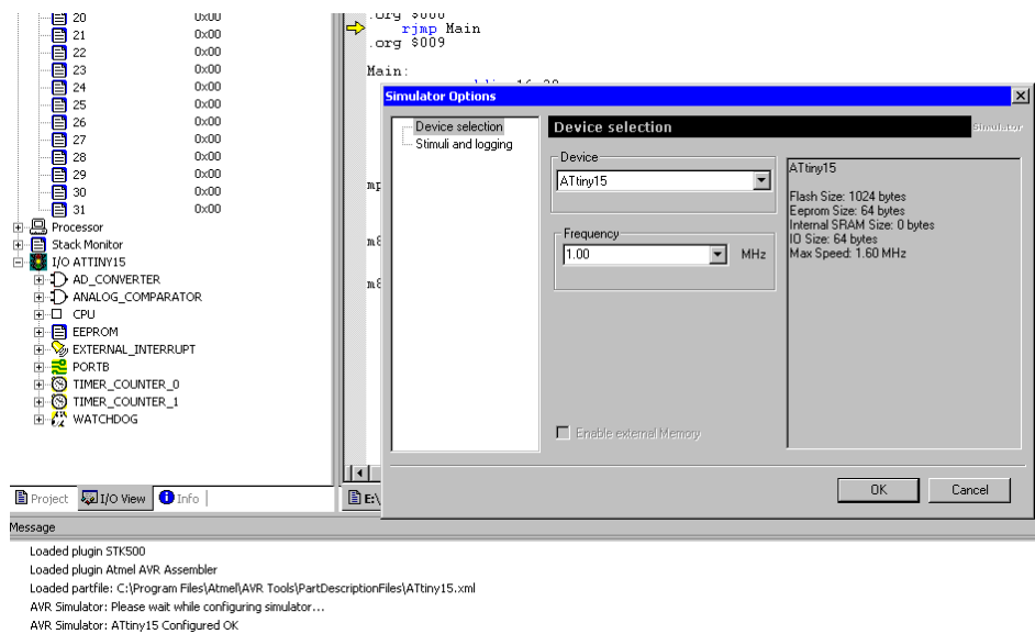
Рисунок 5.8 – Встановлення частоти роботи мікроконтролера
