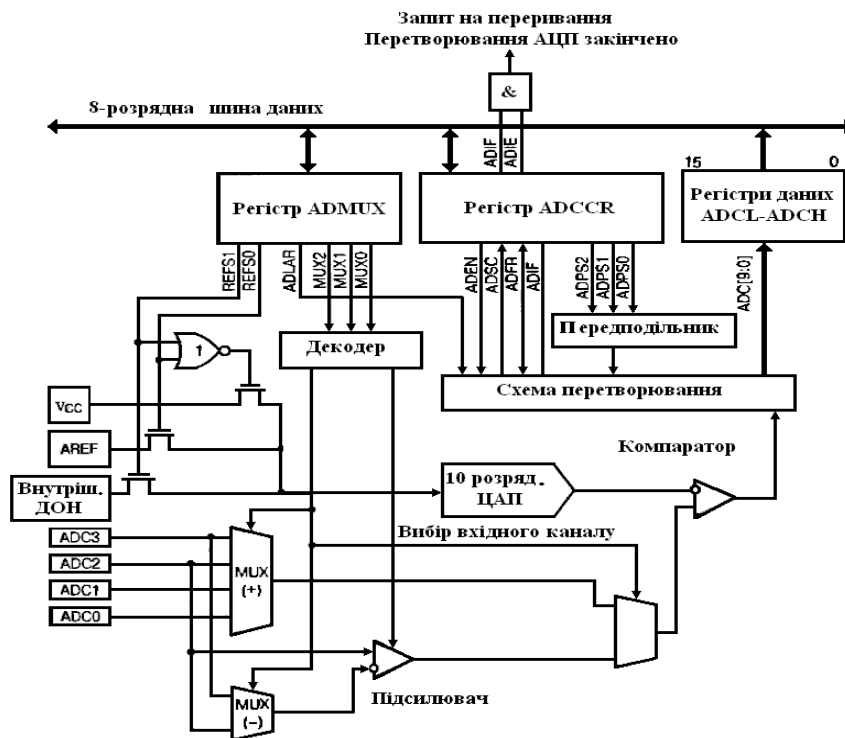
Рисунок 12.2 – Структурна схема АЦП
