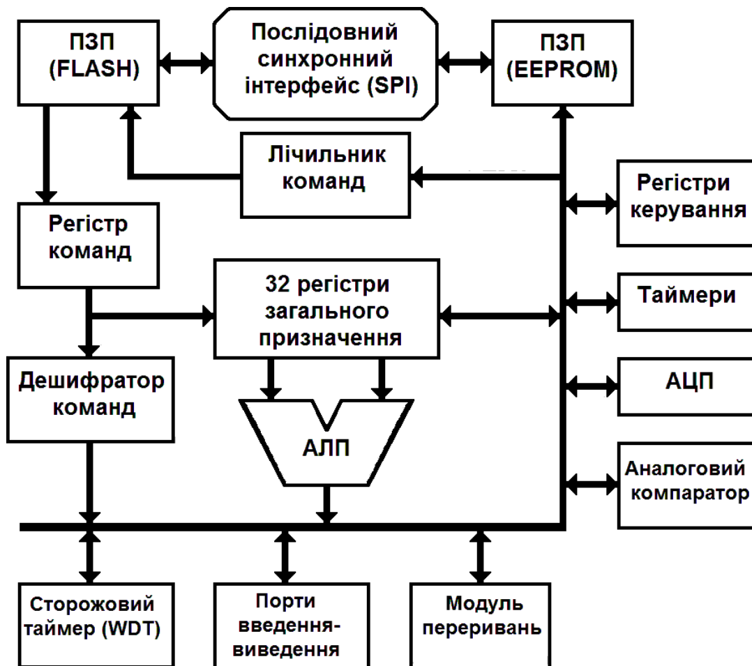
Рисунок 2.1 – Структурна схема мікроконтролера ATtiny15L
