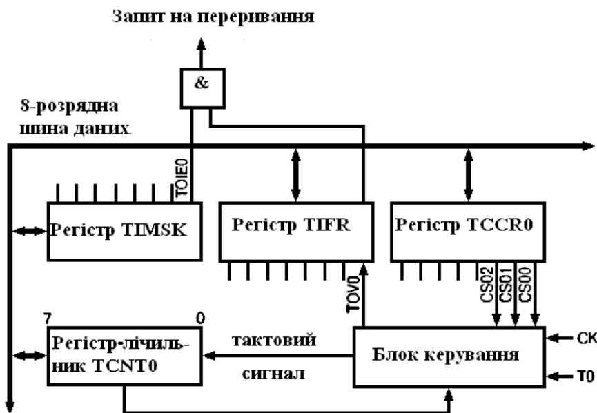
Рисунок 11.1 – Структурна схема таймера T0
