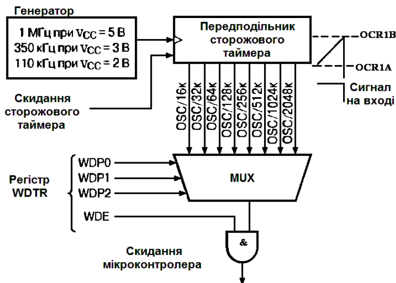
Рисунок 11.5 – Структурна схема сторожового таймера
