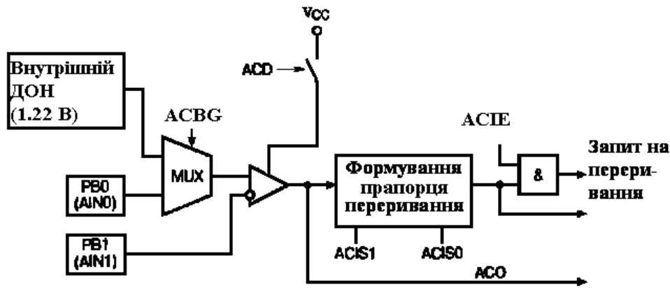
Рисунок 12.1 – Структурна схема аналогового компаратора
