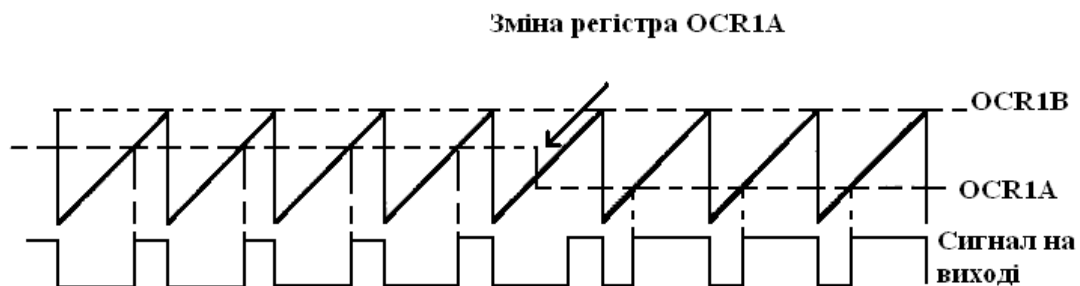
Рисунок 11.4 – Формування ШІМ-сигналів
