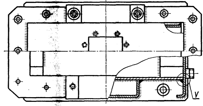
Фиг. 2. Корпус червячного редуктора, выполненный из тонкостенных элементов
