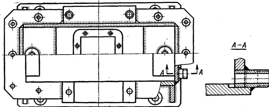
Фиг. 1. Корпус червячного редуктора
