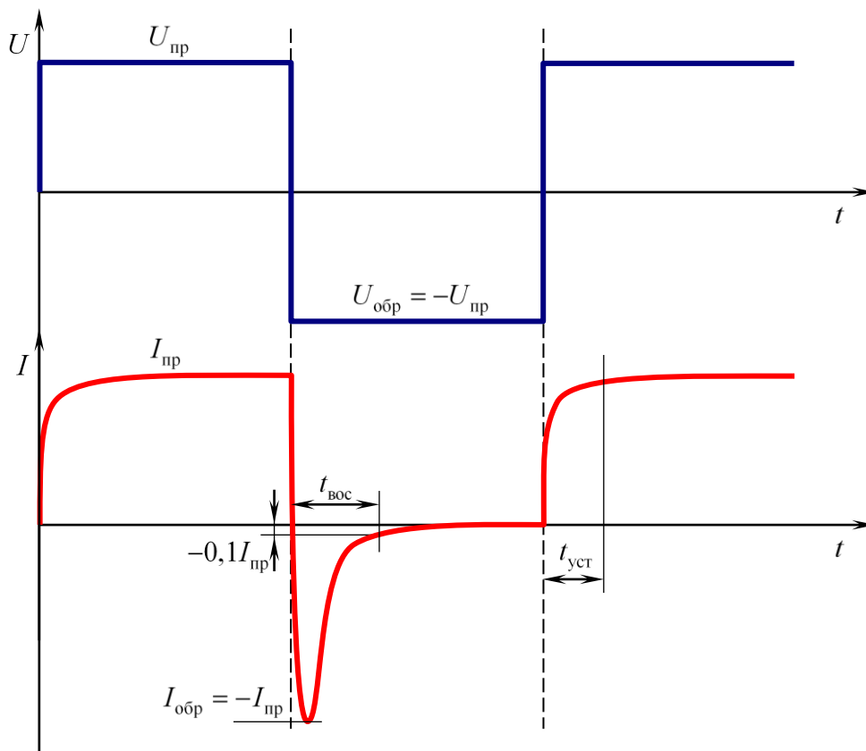
Рис.10.6. Переходные процессы в p-n переходе
