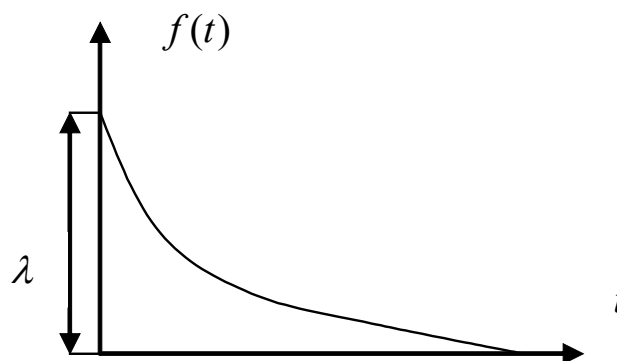
Рисунок 4.2 – Залежність щільності імовірності відмови від часу
