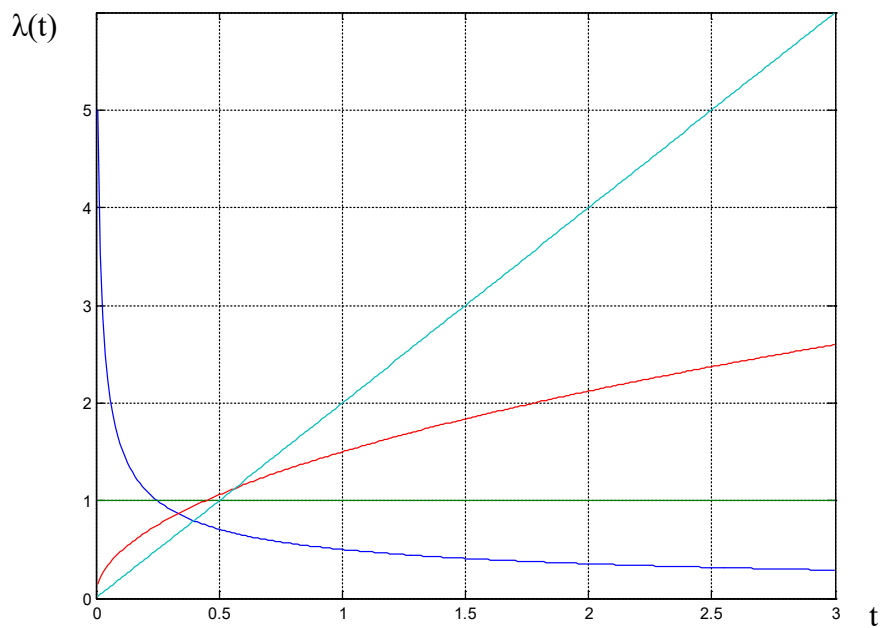
Рисунок 4.6 – Графік інтенсивності відмов, при різних значеннях b
