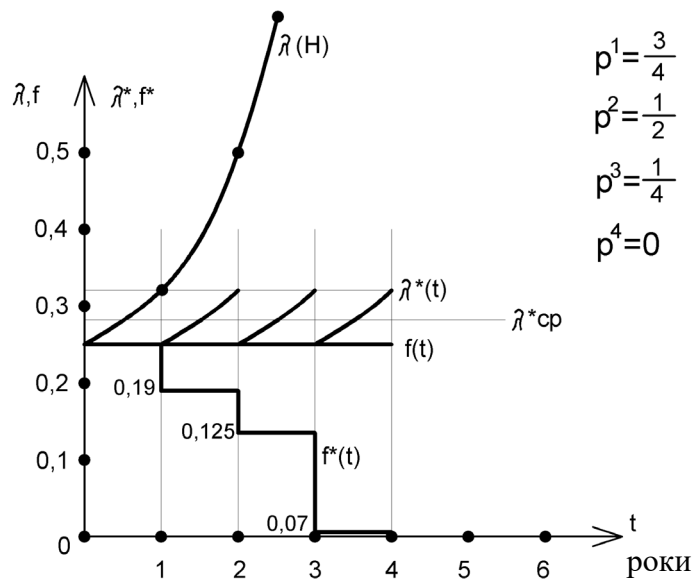
Рисуюнок 12.1 – Графіки залежностей f(t) , \lambda(t) , f^*(t) , \lambda^*(t) від часу
