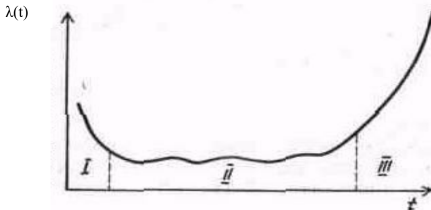
Рисунок 6.2 – Залежність інтенсивності відмов від часу
