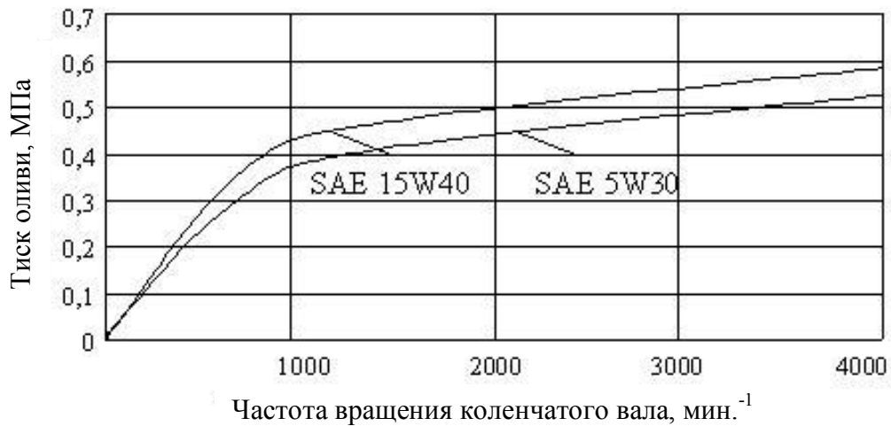
Рисунок 2 – Изменения давления в системе смазки от частоты вращения коленчатого вала при постоянной температуре 65°С
