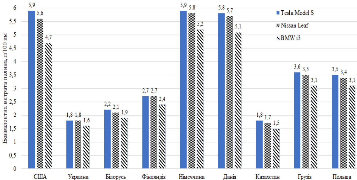
Рисунок – Результати розрахунку еквівалентної витрати палива Tesla S, Nissan Leaf та BMW i3 при їх експлуатації у різних країнах
